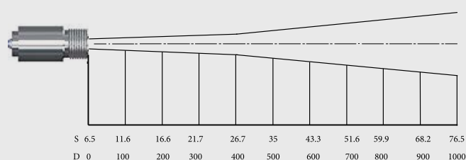
SF optics, D:S = 15:1
